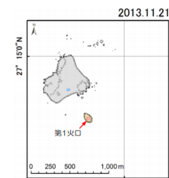
調査結果の概略図 (基図: 海図W1356「西ノ島」)
